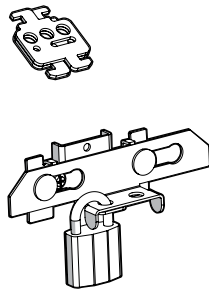
Mechanical padlock apparatus Aparato de bloqueo de la suspensión mecánica
